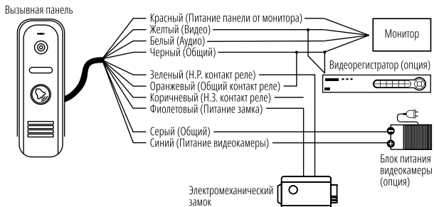
Схема подключения вызывной панели MASK к электромеханическому замку без блока питания
