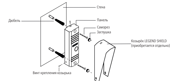
Рис. 9 Фронтальная установка вызывной панели
