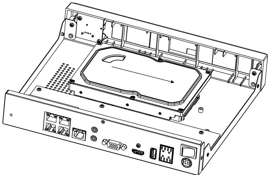
Рис. 16. Установка жесткого диска
