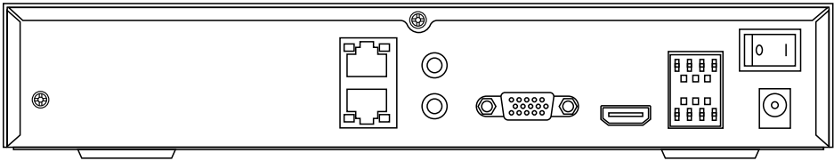
Рис. 8. Задняя панель NR1808X | NR2816X
