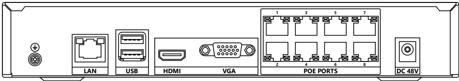
Рис. 6. Задняя панель NR1608X-P8
