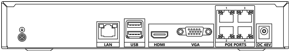
Рис. 5. Задняя панель NR1604X-P4
