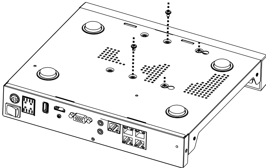
Рис. 17. Установка жесткого диска
