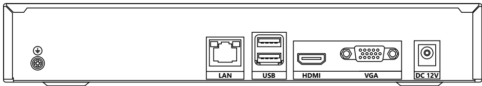
Рис. 4. Задняя панель NR1604X | NR1608X | NR1616X
