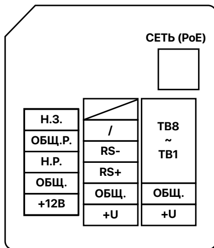
Рис. 7 Проводные интерфейсы видеодомофона
