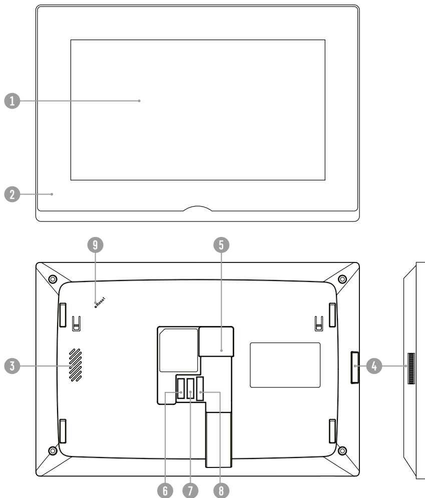
Рис. 2 Видеодомофон IMPULSE
